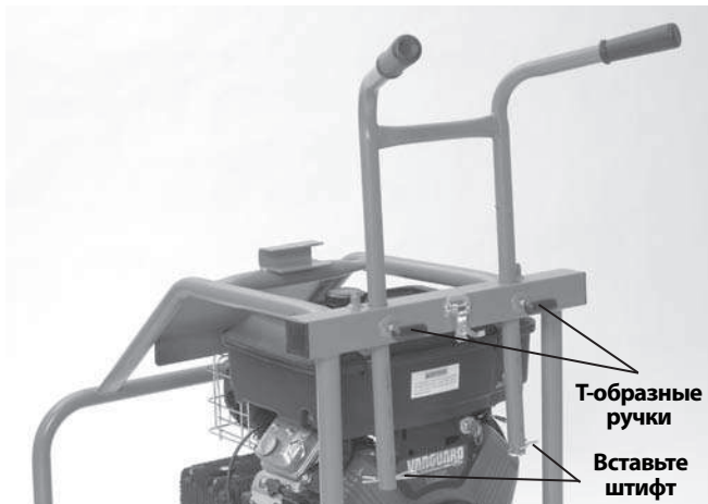
Рис. 5 – Сборка рукоятки KJ-3100
